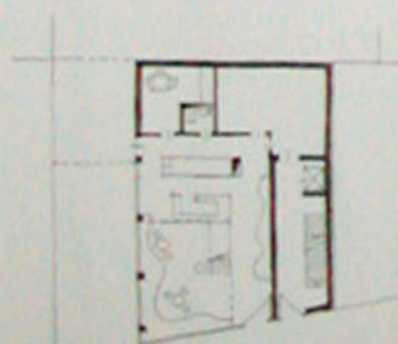
BA 1000 Galerie Laden
