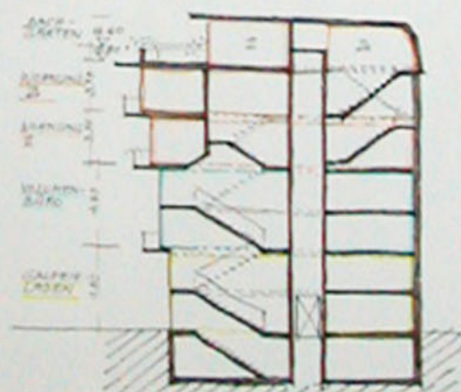
SCHNITT DURCH DAS TREPPENHAUS M 1:100
