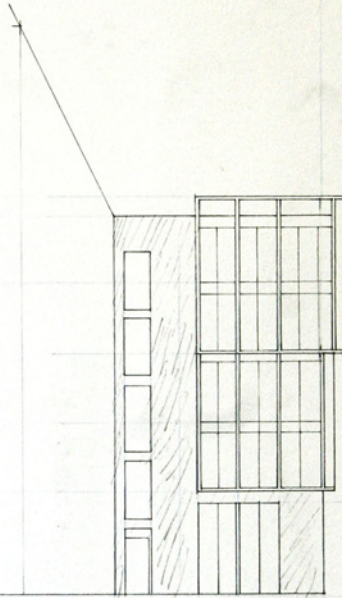
ANSICHT NORD M 1:100
